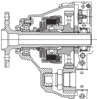
Bild 7 02531 HINWEIS: Bild zeigt ein Getriebe „Ausführung 2“ mit integrierter Überlastkupplung.
